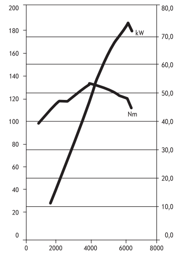
Drehmoment (Nm) 1.4 TWINPORT 74 kW Leistung (kW)
