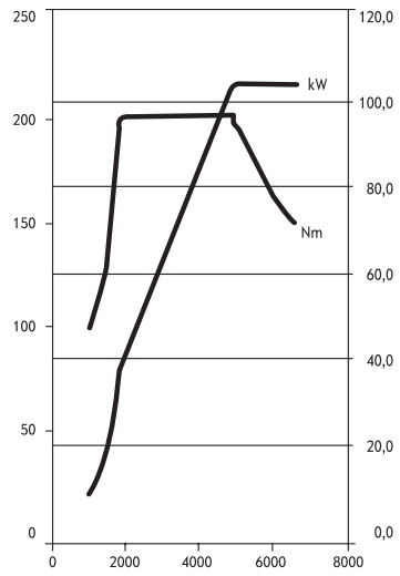
Drehmoment (Nm) 1.4 TURBO 103 kW Leistung (kW)
