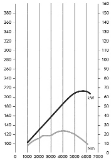
Drehmoment (Nm) 1.4 TWINPORT 64 kW Leistung (kW)
