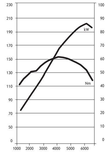
Drehmoment (Nm) 1.6 DOHC 85 kW Leistung (kW)
