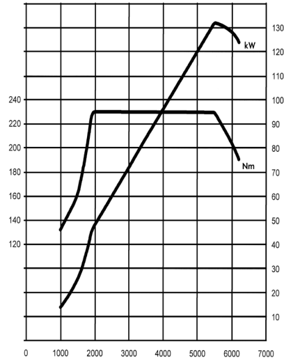
Drehmoment (Nm) 1.6 TURBO 132 kW Leistung (kW)
