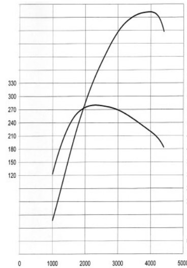
Drehmoment (Nm) 1.7 CDTI 92 kW Leistung (kW)
