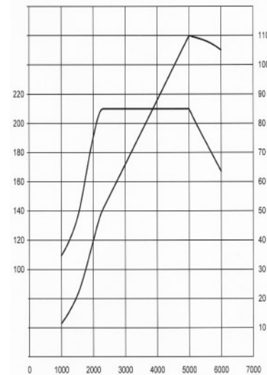
Drehmoment (Nm) 1.6 Turbo CNG 110 kW Leistung (kW)
