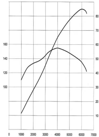
Drehmoment (Nm) 1.6 DOHC 85 kW Leistung (kW)
