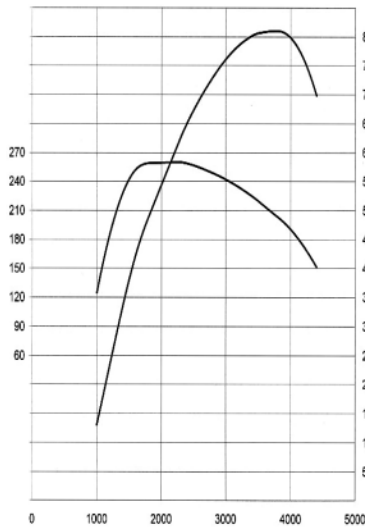
Drehmoment (Nm) 1.7 CDTI 81 kW Leistung (kW)
