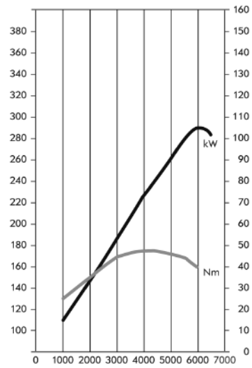
Drehmoment (Nm) 1.8 DOHC 103 kW Leistung (kW)
